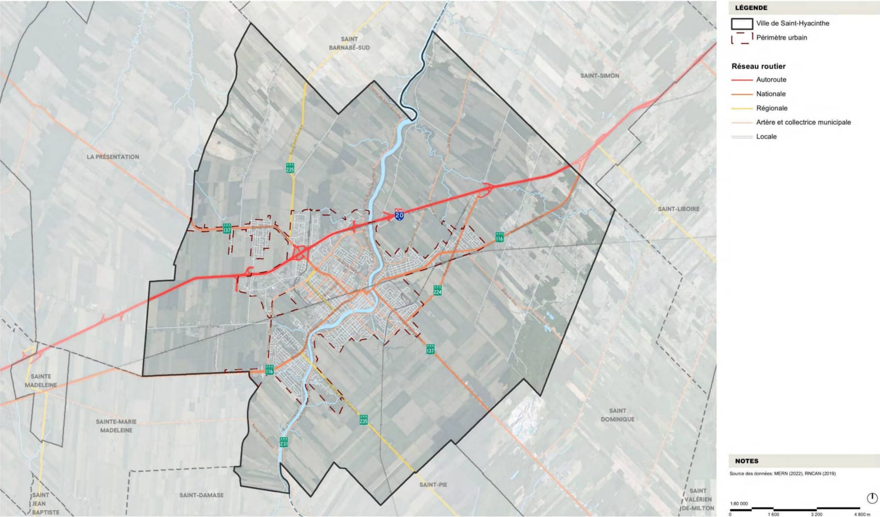
FIGURE 38 - Réseau routier
