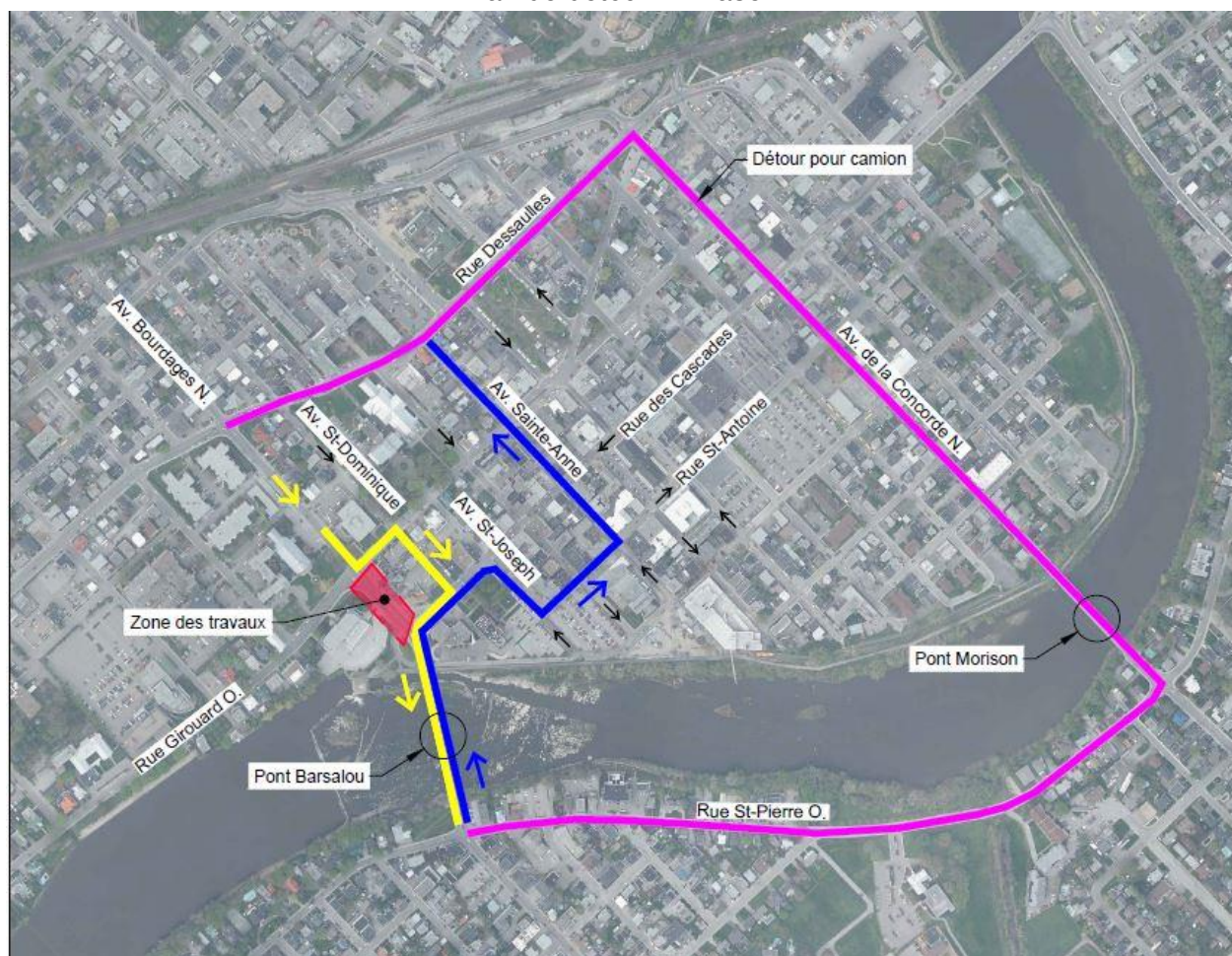
Plan de détour – Phase 1
